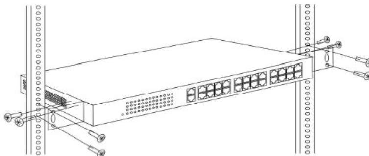
图表 2-1 机架安装示意图
